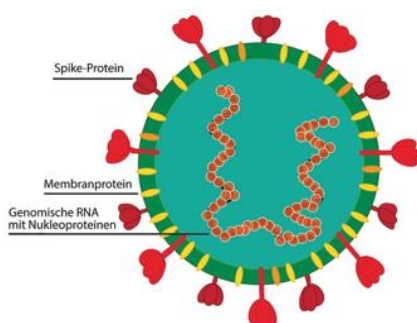
Abbildung 7–1: SARS-CoV-2, schematische Darstellung mit Spike-Protein, Membranprotein und Virus-RNA. Quelle: Witt et al. 2020 https://doi.org/10.1002/ciuz.202000058
